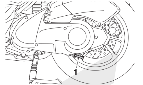
۱. V-belt case check hose
